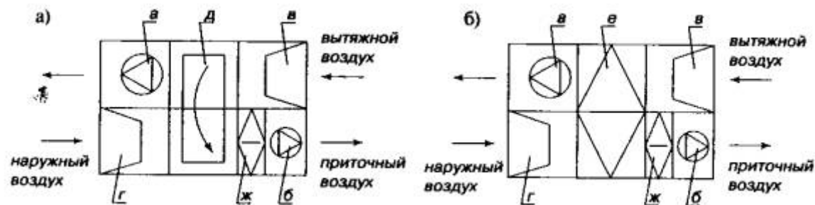
Рис. 8. Утилизаторы тепла вытяжного воздуха:
