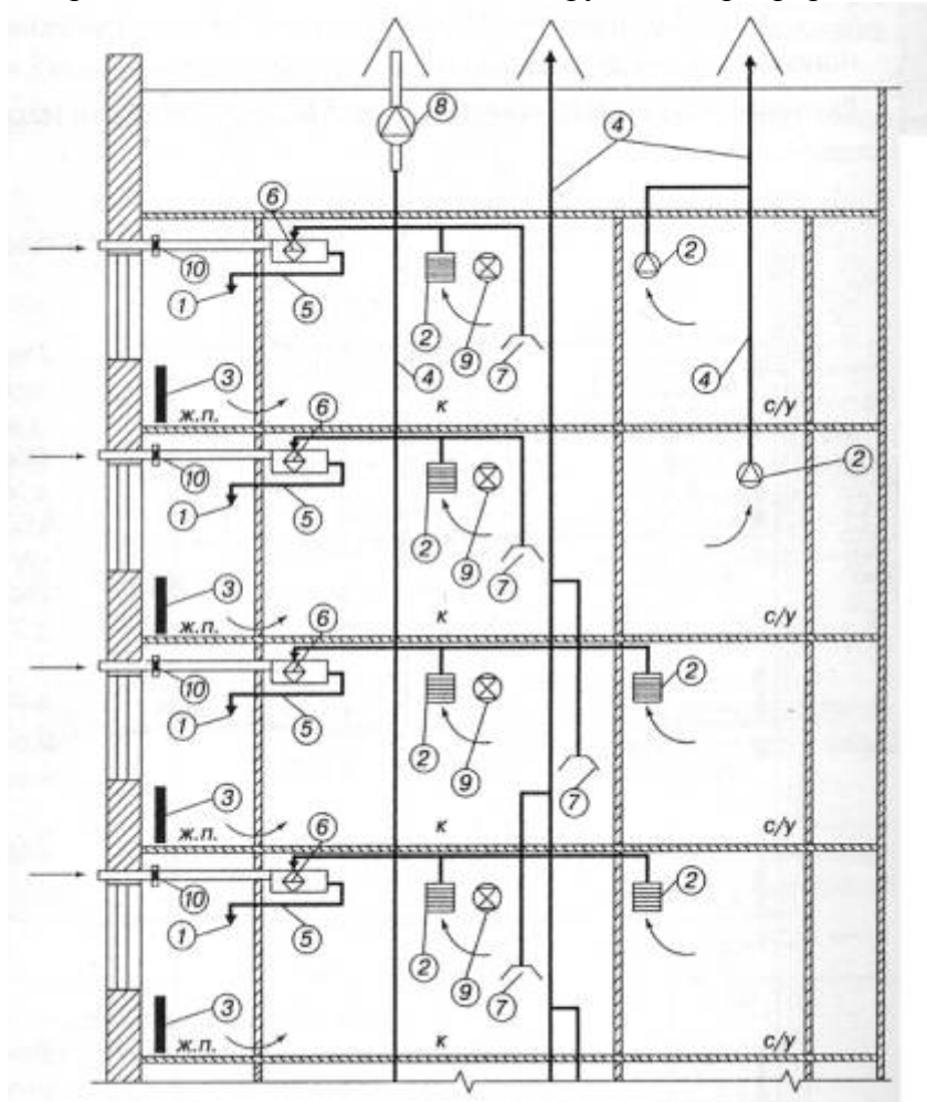
Рис. 6. Схема системы механической приточно-вытяжной вентиляции с утилизацией тепла вытяжного воздуха (индивидуальный утилизатор). Обозначения:
