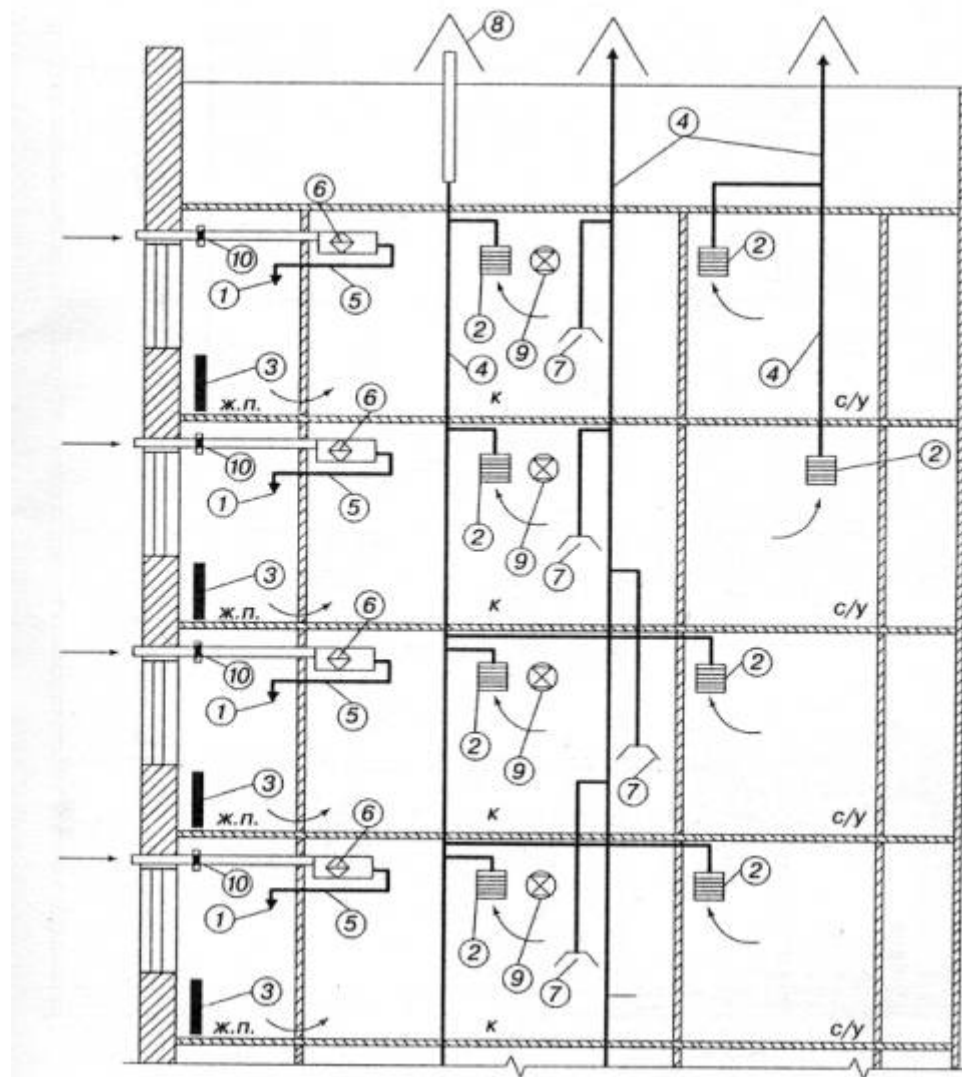
Рис. 5. Схема системы механической приточной вентиляции с естественным удалением воздуха.
