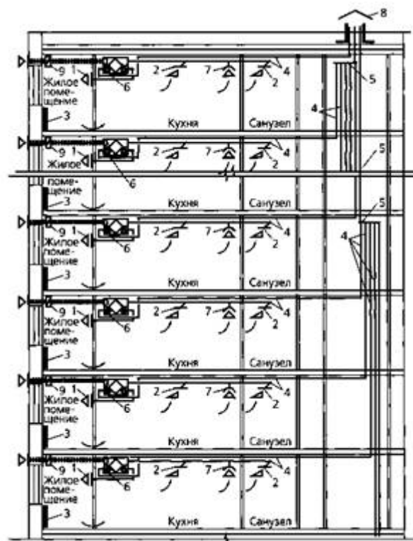
Рисунок 10 - Схема системы механической приточно-вытяжной вентиляции (децентрализованной) с утилизацией теплоты удаляемого воздуха:
